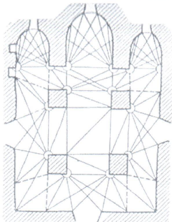
Рисунок Б.1 — Схема обмера плана методом триангуляции
