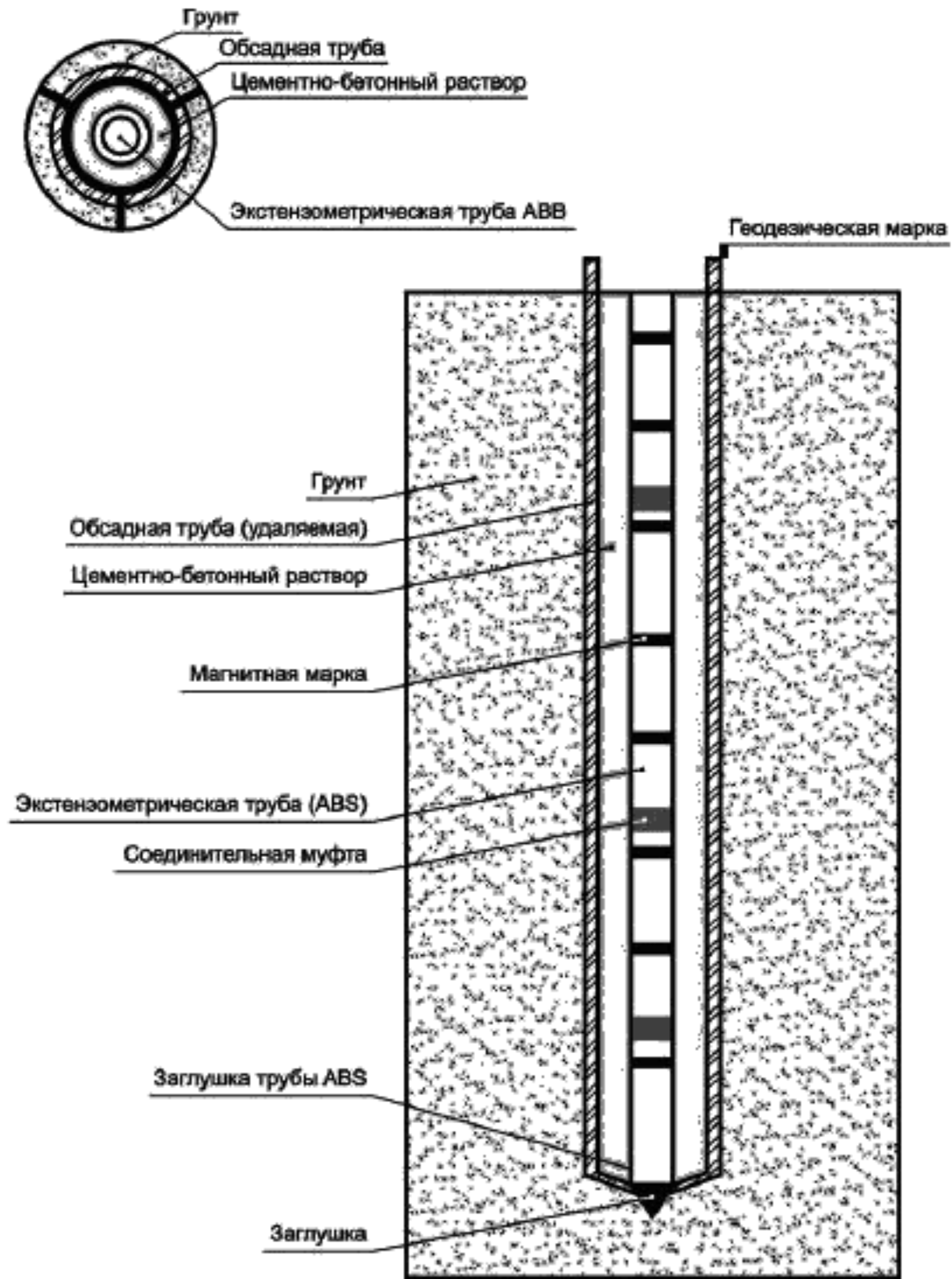
Рисунок Д.2 — Схема экстензометрической наблюдательной скважины
