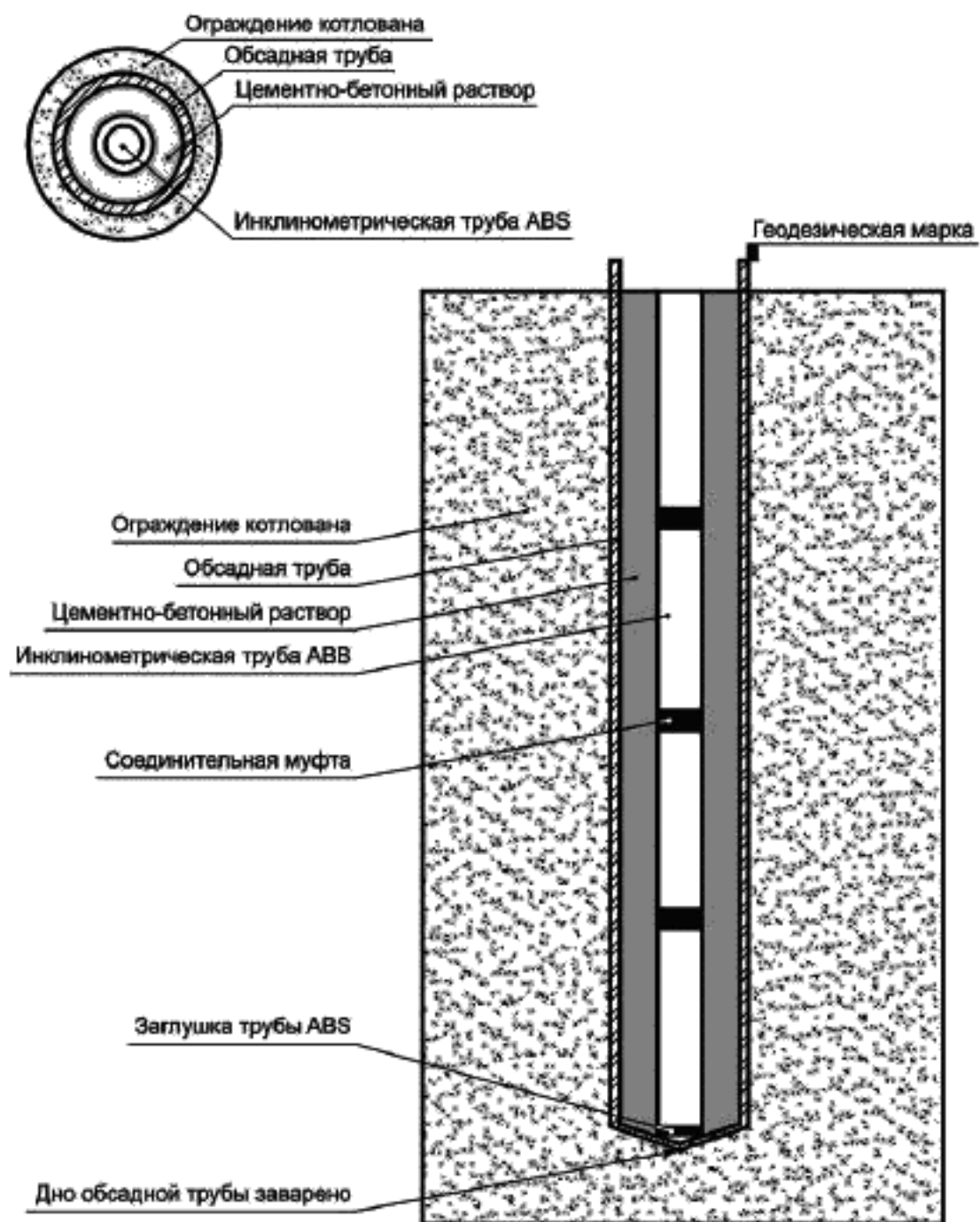
Рисунок Д.1 — Схема инклинометрической наблюдательной скважины
